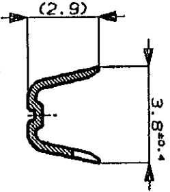
断面 C-C SECT. C-C
