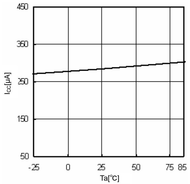
Fig.10 T a -I cc
