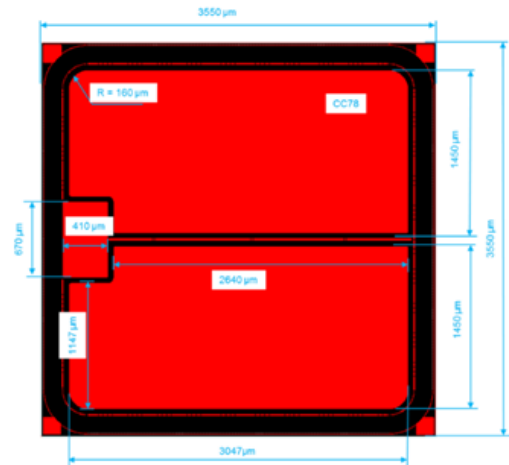
DIE OUTLINE
