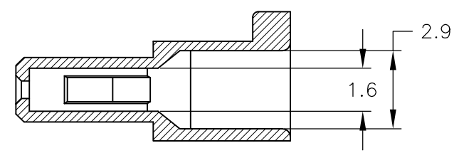
断面 A-A
