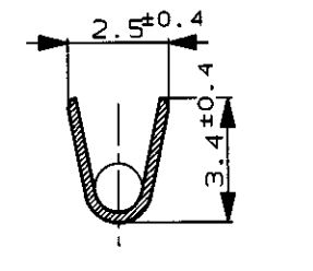
断面 C-C (SECT. C-C)
